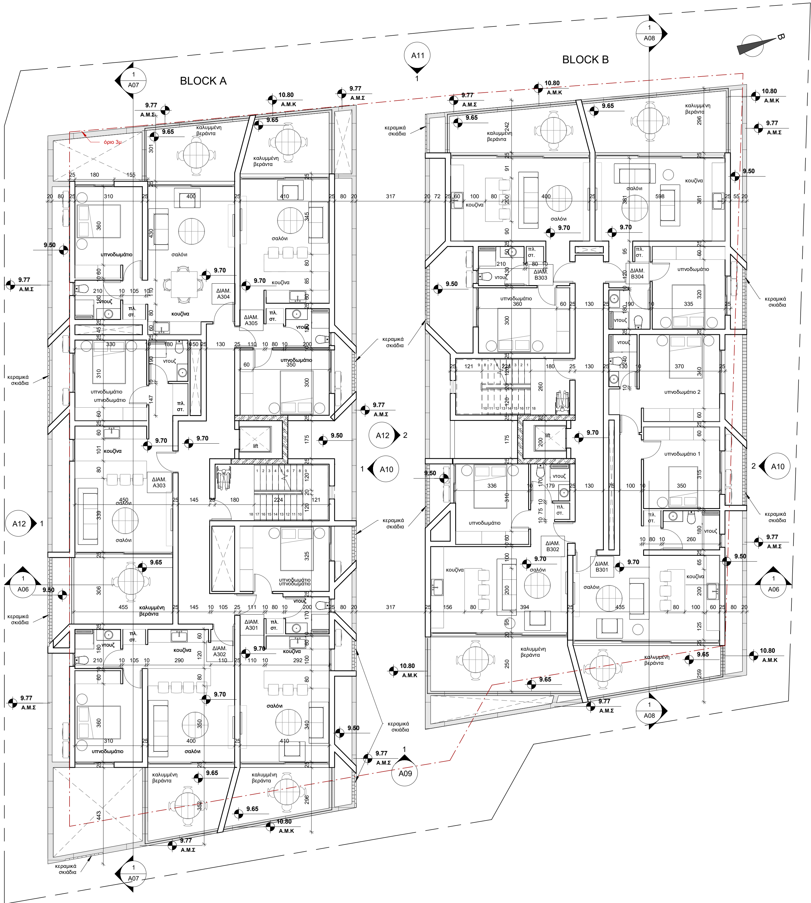
1 04 - Κάτοψη 3ου Ορόφου 1: 100
