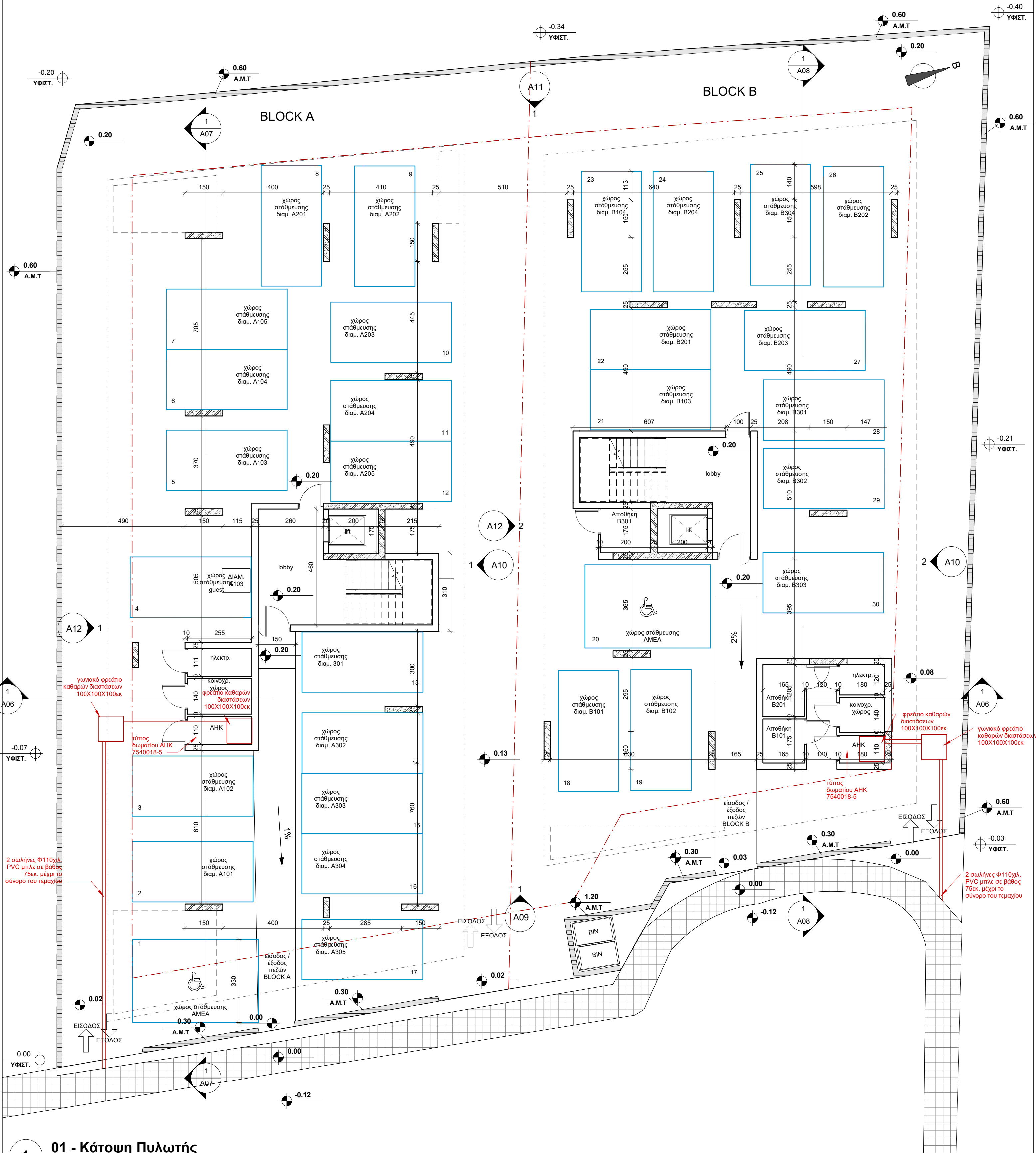
1 01 - Κάτοψη Πυλωτής 1 : 100
