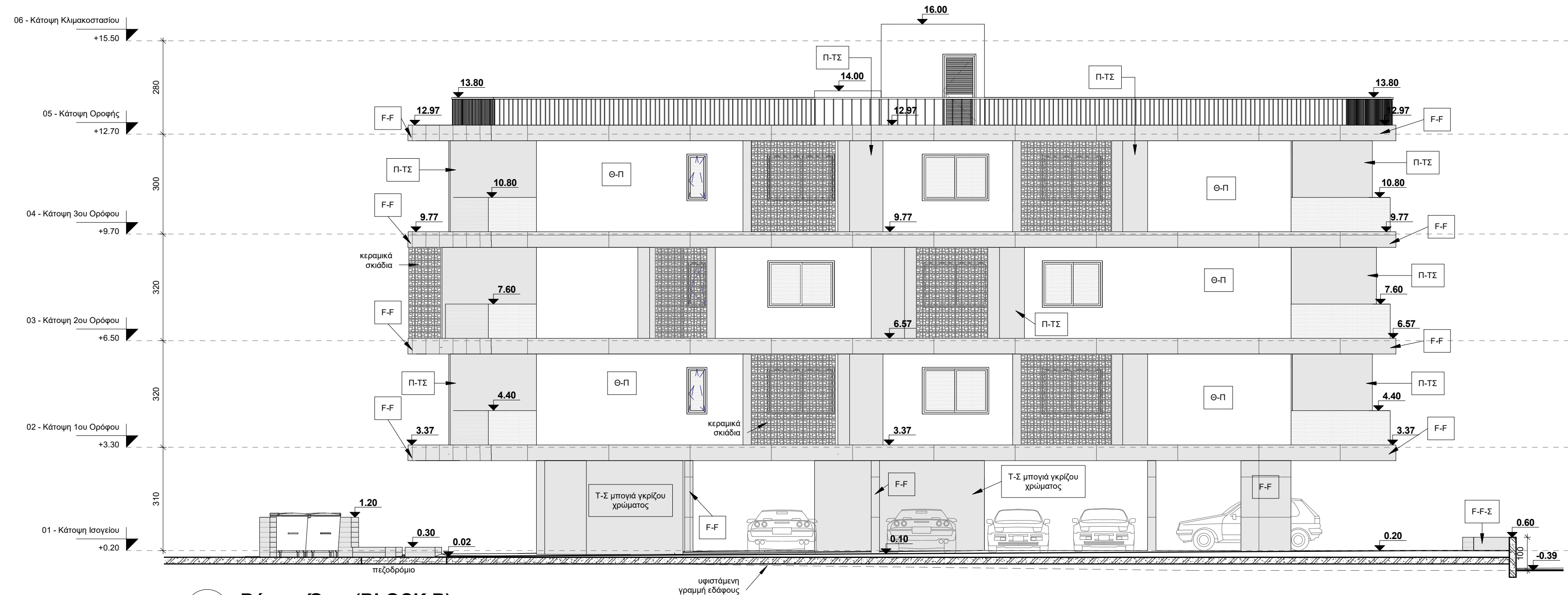
Βόρεια Όψη (BLOCK B) 1 : 100
