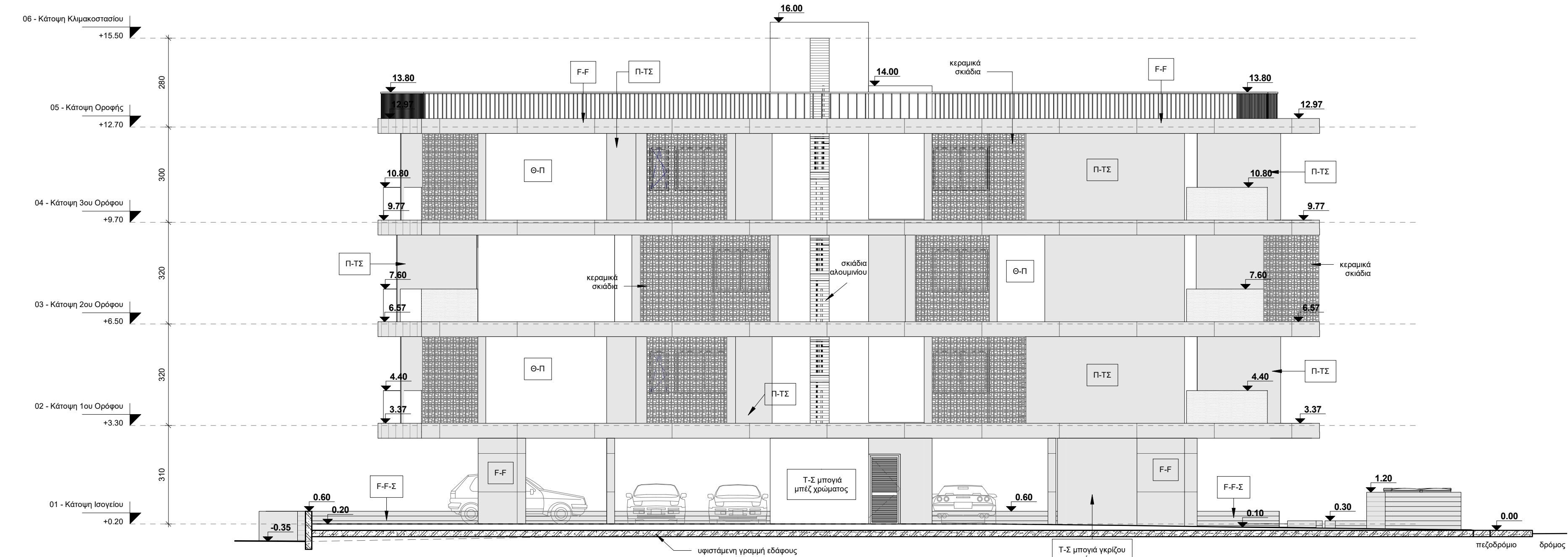
2 Νότια Όψη (BLOCK B) 1 : 100
