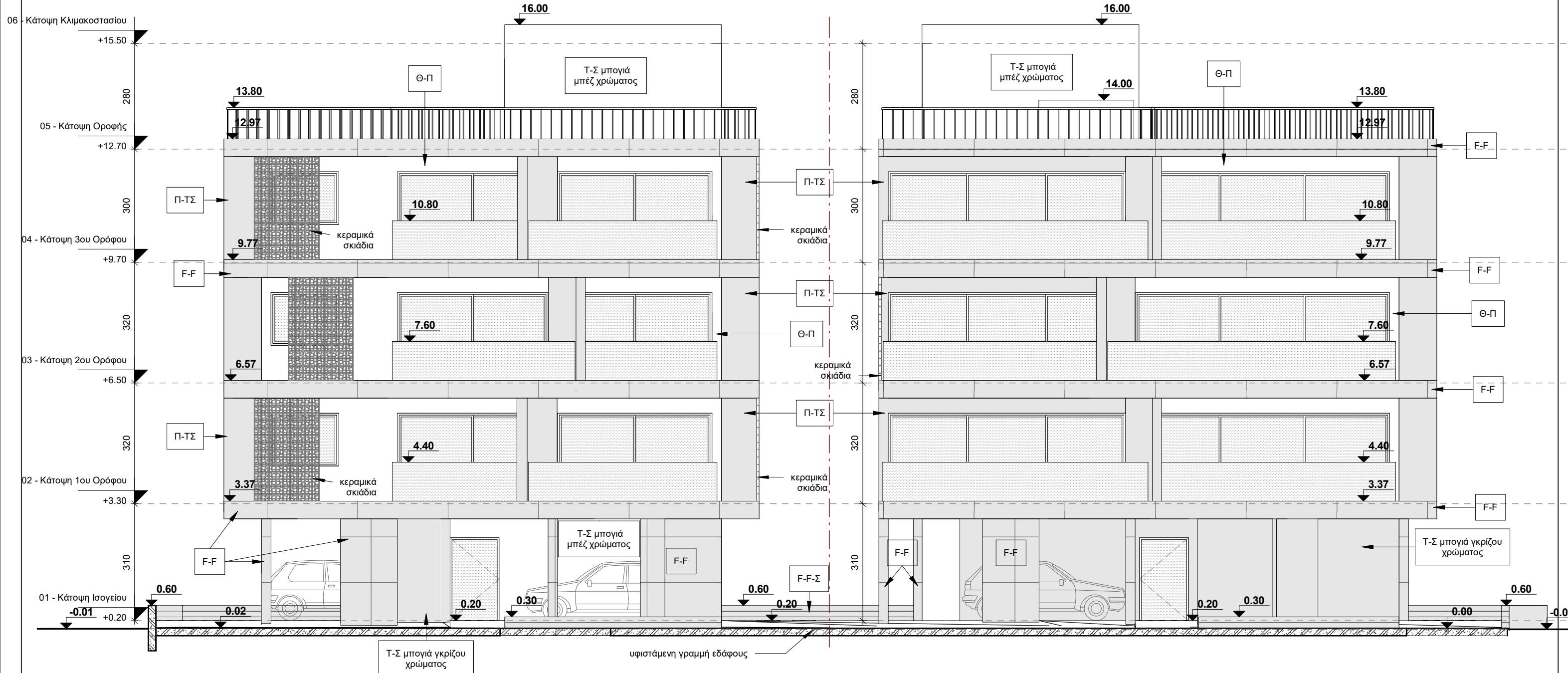
1 Ανατολική Όψη 1 : 100
