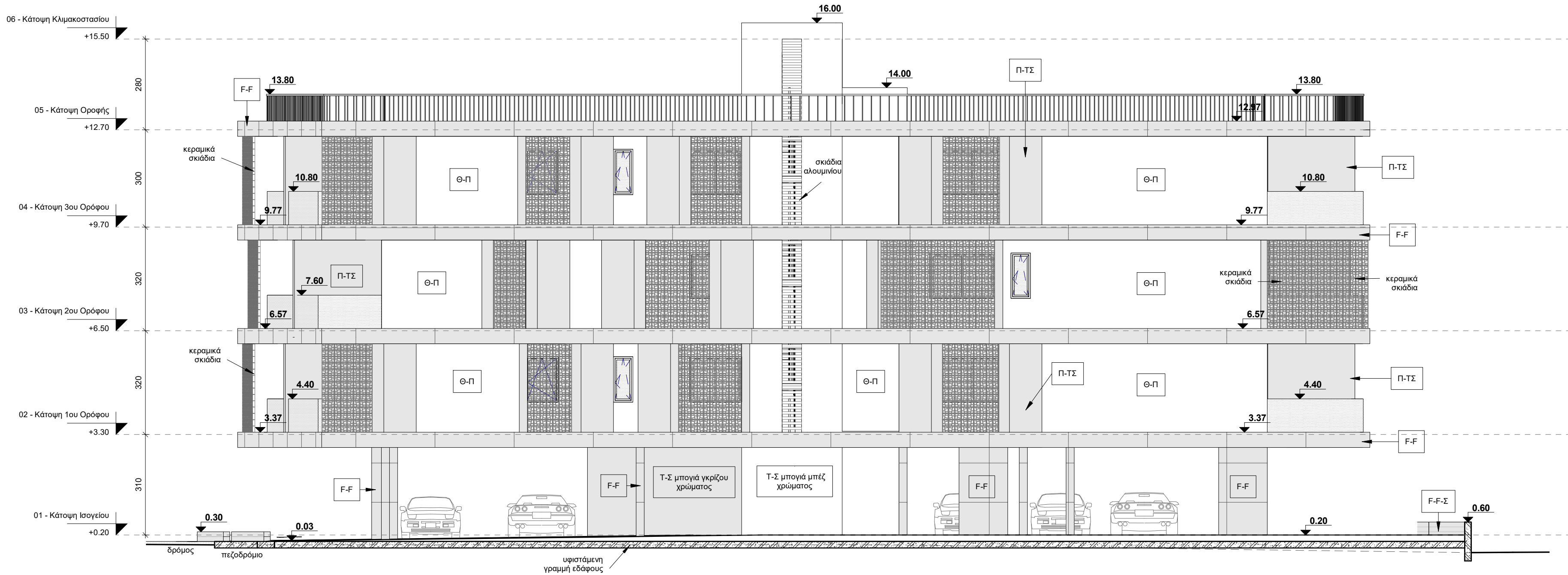
Βόρεια Όψη (BLOCK A) 1 : 100
