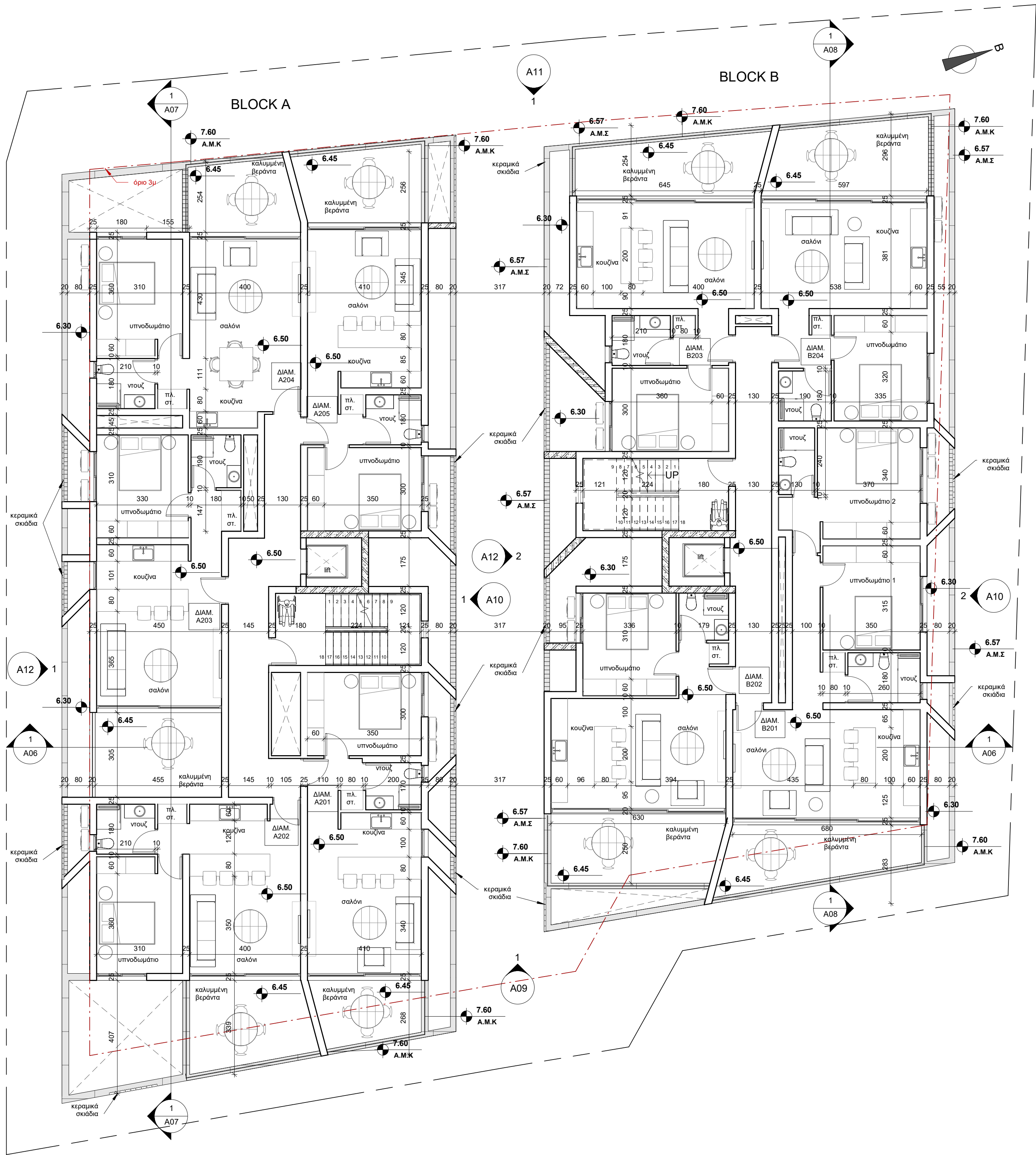
1 03 - Κάτοψη 2ου Ορόφου 1 : 100
