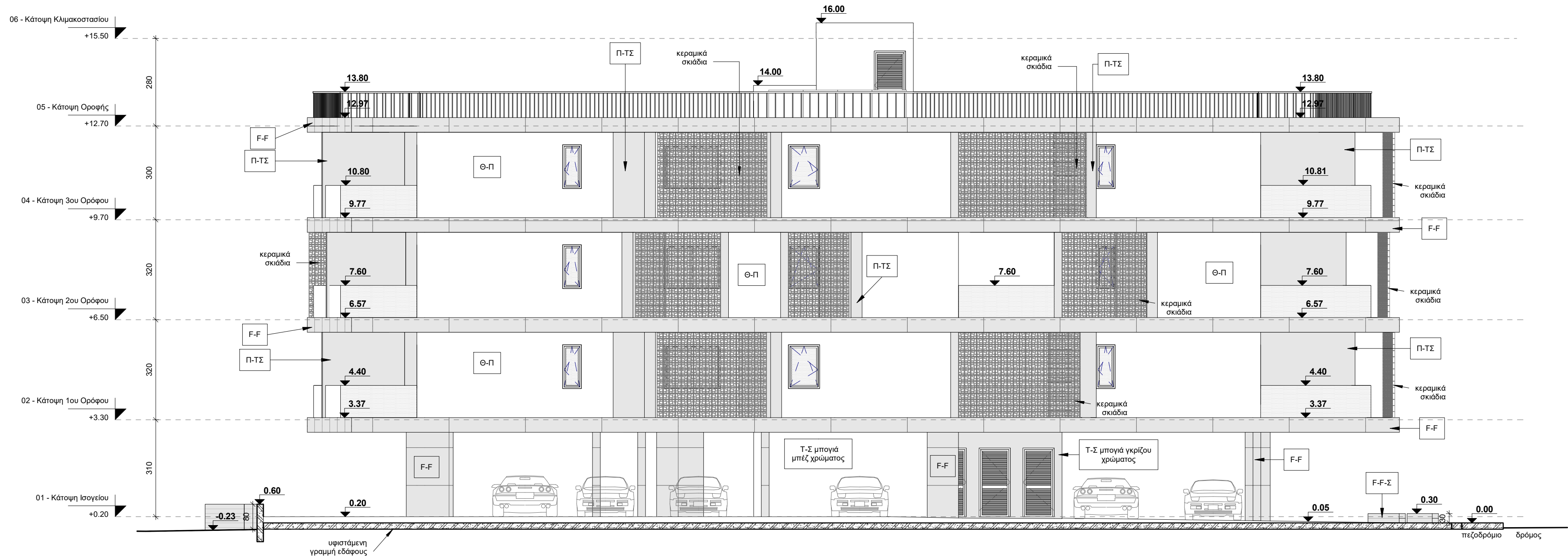
1 Νότια Όψη (BLOCK A) 1 : 100
